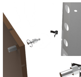
Sistema di aggancio rapido Quick hooking system
